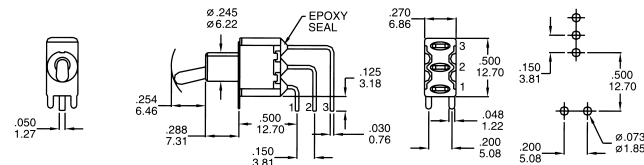
SPDT
